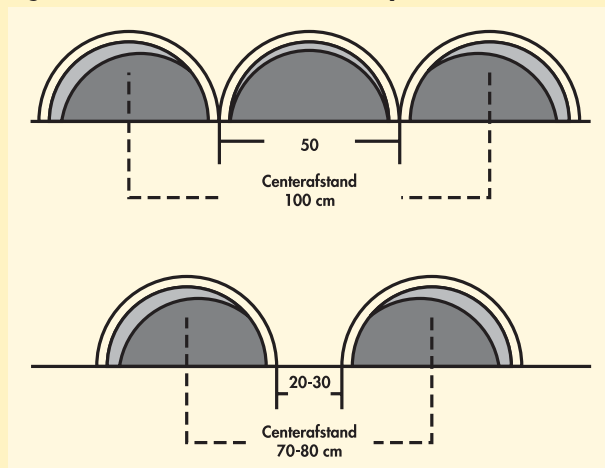
Figur 1. Skitse af rundbuekanal system (G900)
